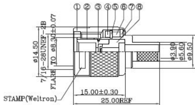
(RG59U, RG62U)
