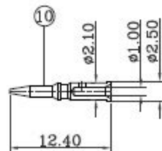
(RG59U-PLENUM)
